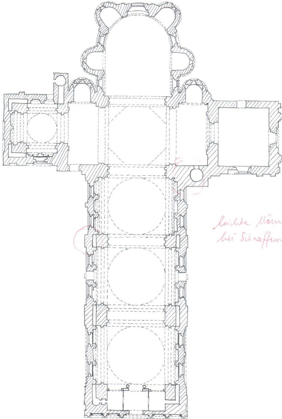
KATHEDRALE SAINT-PIERRE, ANGOULEME (F), 1110
