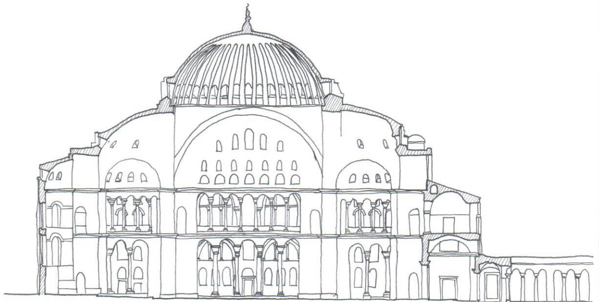
Konstantinopel, Hagia Sophia. 532-537
