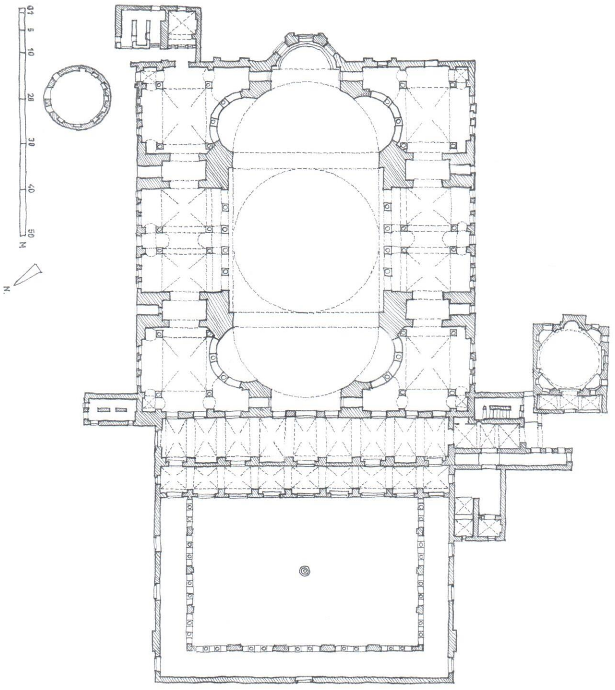
Konstantinopel, Hagia Sophia, 532-537.
