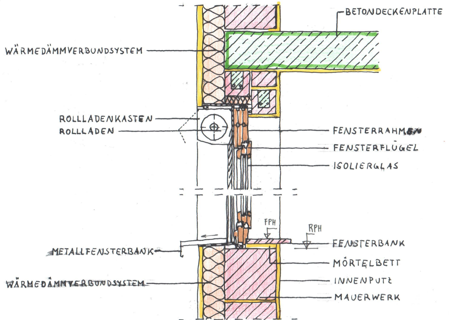
FENSTER IN MAUERWERK MIT WDV-S-DÄMMUNG UND AUSSENLIEGENDEM ROLLADENKASTEN LOTSCHNITT STANDARD-DETAIL M-1:10
