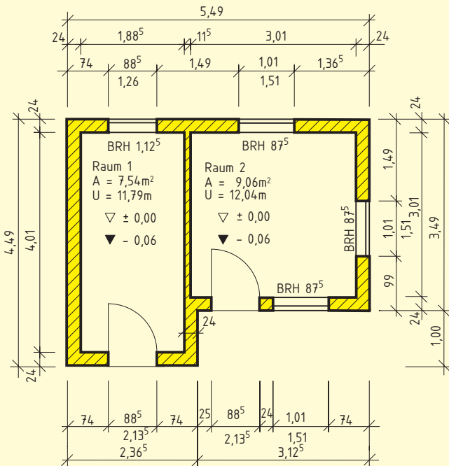
Ausführungszeichnung (Grundriss)
