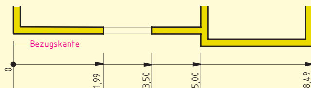
Bezugsbemaßung in steigender Bemaßung
